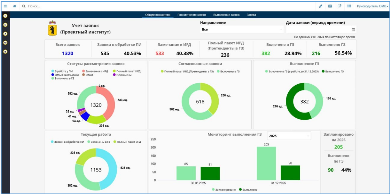
Рисунок 5 – Дашборд
